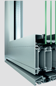
Einsatzfüllung
